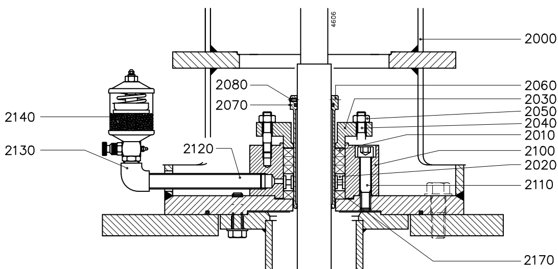
Рисунок 8. Сальниковое уплотнение S3
