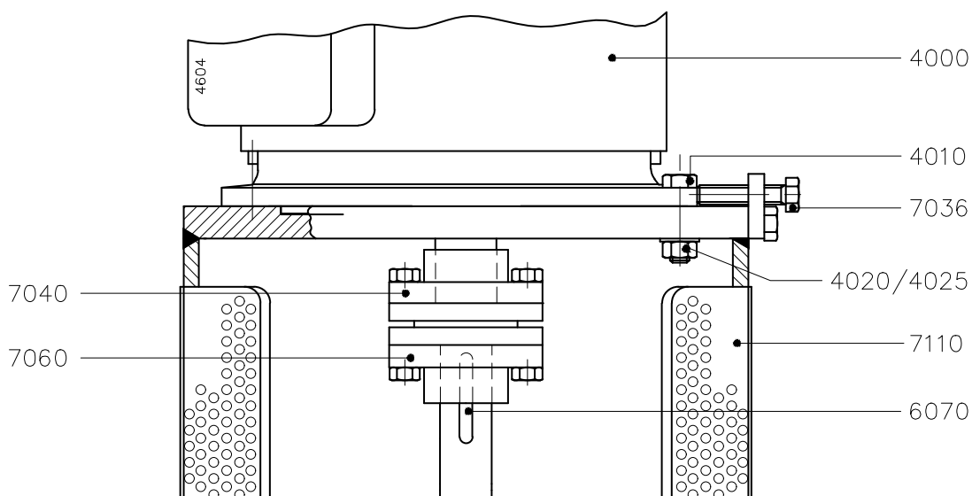
Рисунок 6. Разборка электродвигателя
