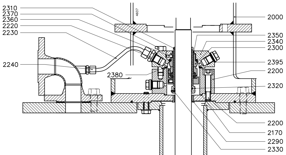
Рисунок 9. Механическое уплотнение M2
