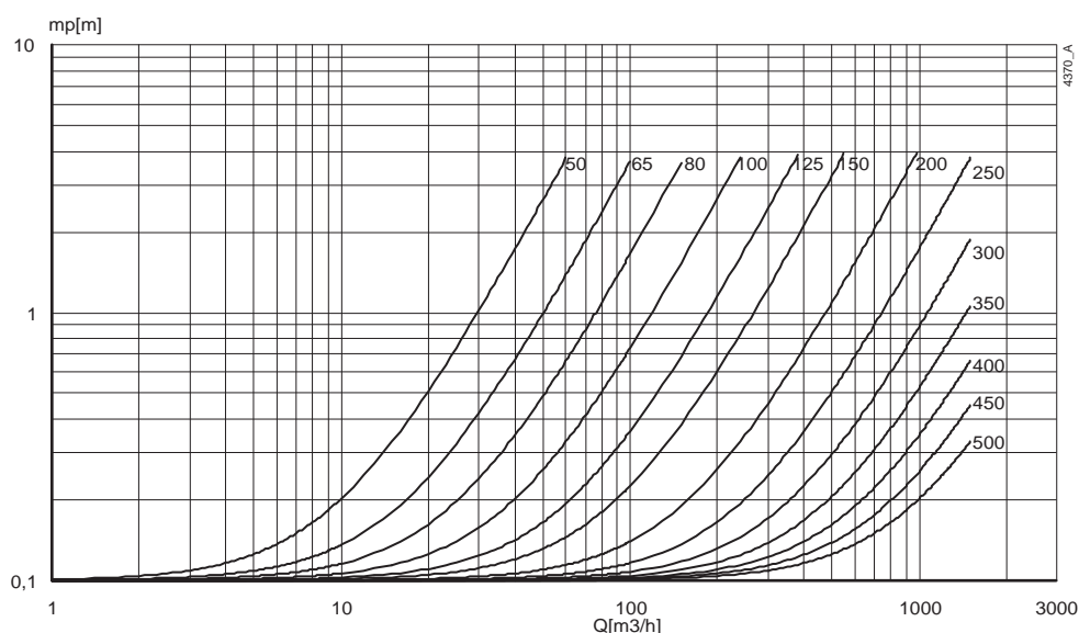
Рисунок 19. Наименьший уровень жидкости в зависимости от производительности и входного диаметра
