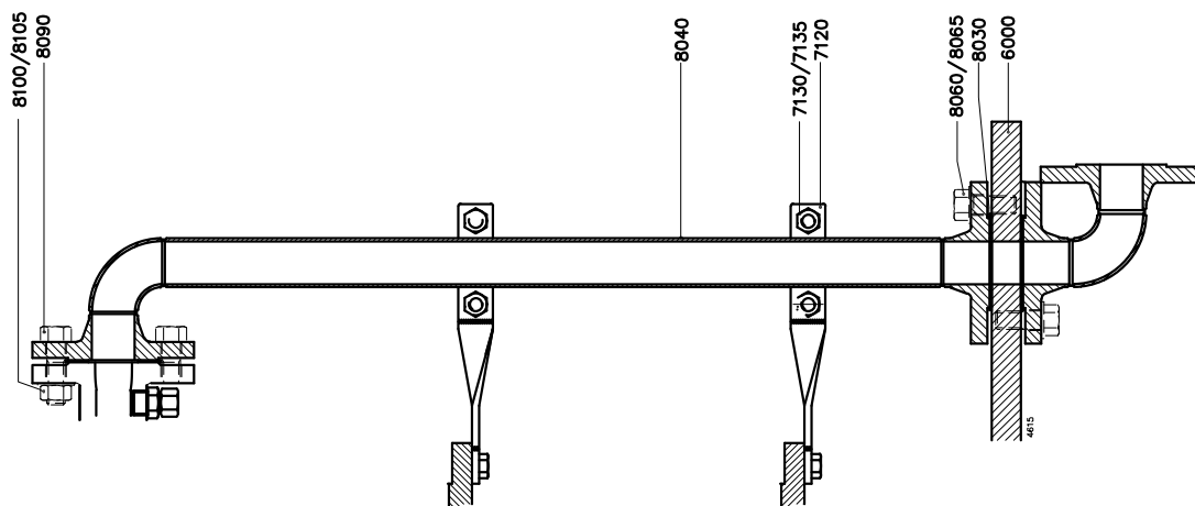
Рисунок 5. Разборка нагнетающего трубопровода
