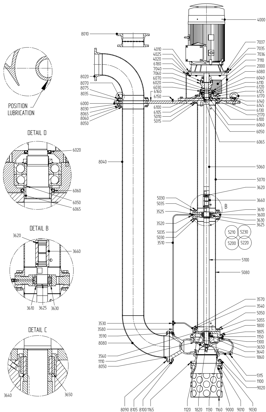
Рисунок 18. Насос с группой уплотнения вала S0, группа кронштейнов подшипников 4
