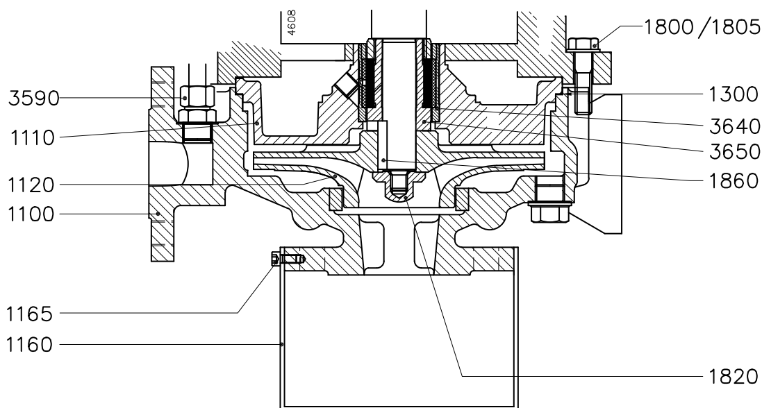
Рисунок 10. Корпус насоса / крыльчатка
