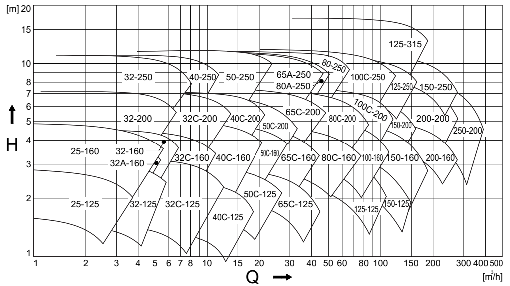
Рисунок 22: Обзор рабочих параметров при 1000 мин -1 .
