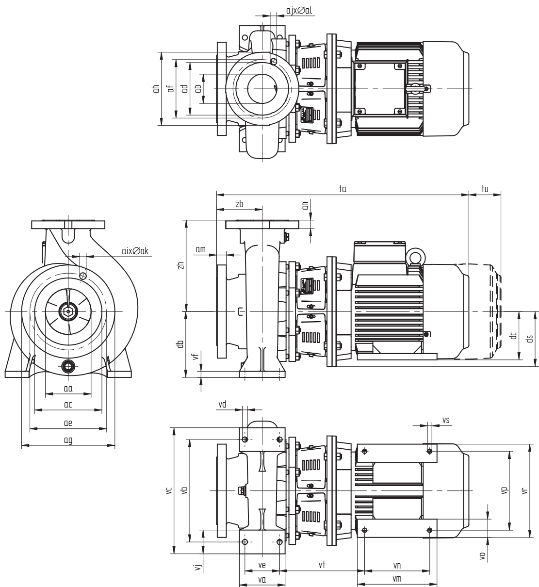
Рисунок 16: Размеры насоса.
